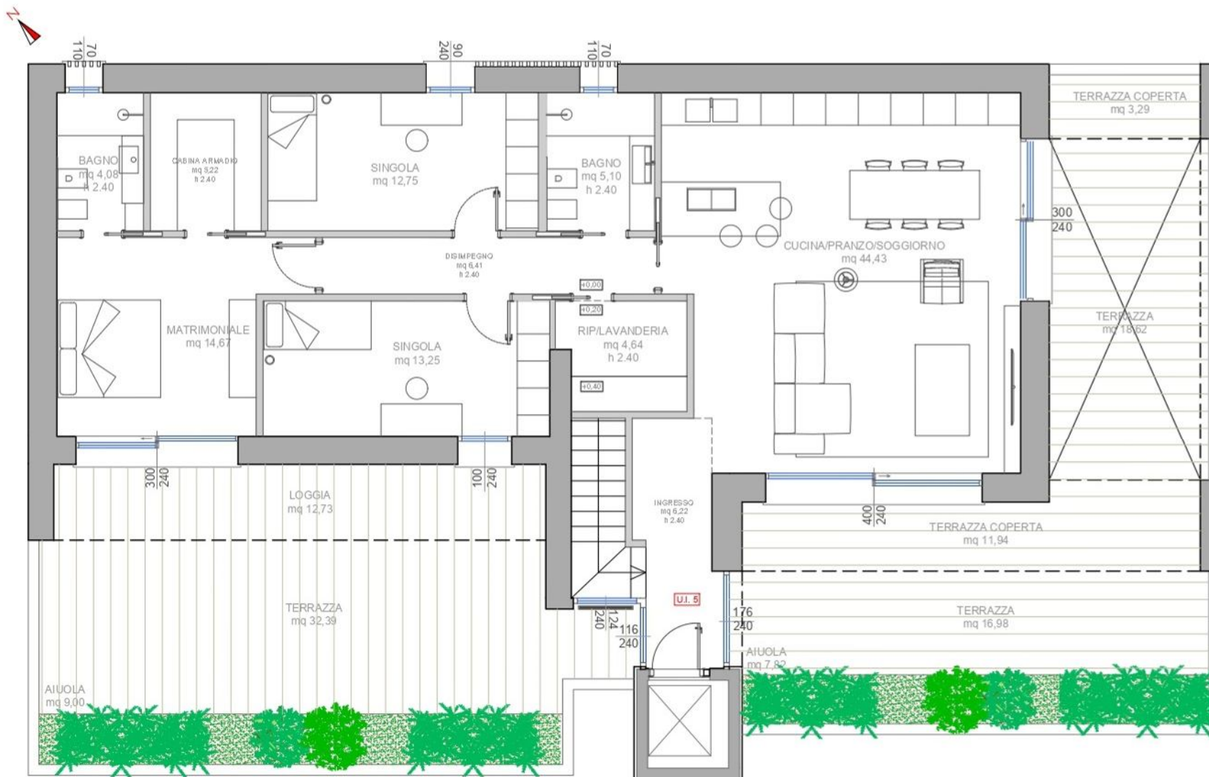
Pianta Attico Piano secondo
