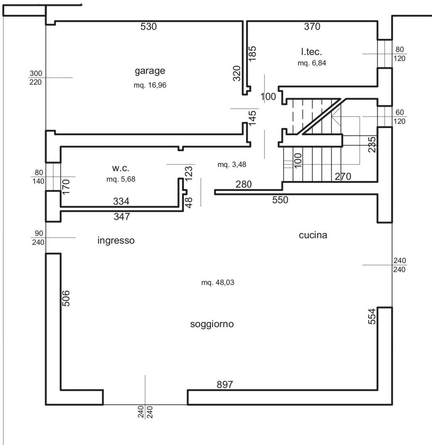
Pianta piano terra 1
